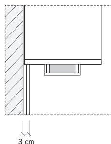
Ponti senza pannello sottoponte Bridging units with no panel underneath
