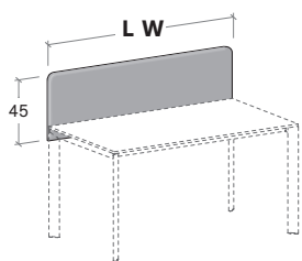
Pannello divisorio Sp. 1,8 cm Partition screen 1,8 cm thick
